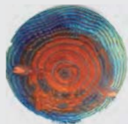
經橫向壓縮處理之 柳杉原木防腐劑滲透圖 (可達k4等級防腐)
