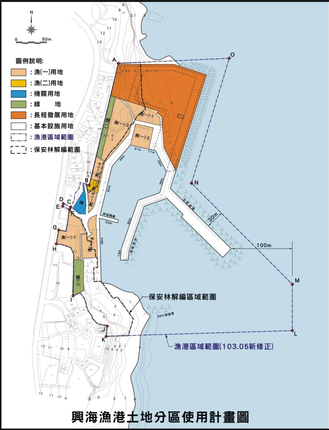
圖 4. 興海漁港土地使用分區計畫圖及使用管制計畫表
